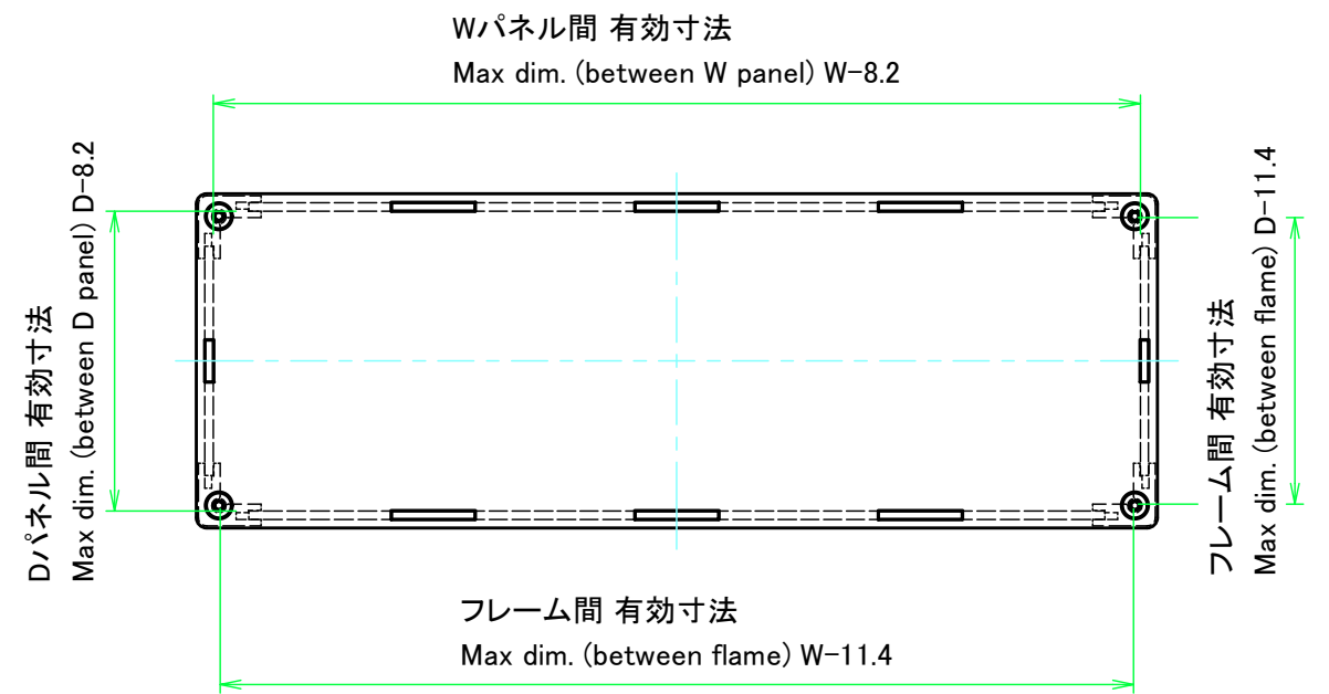
下カバー / Bottom cover
